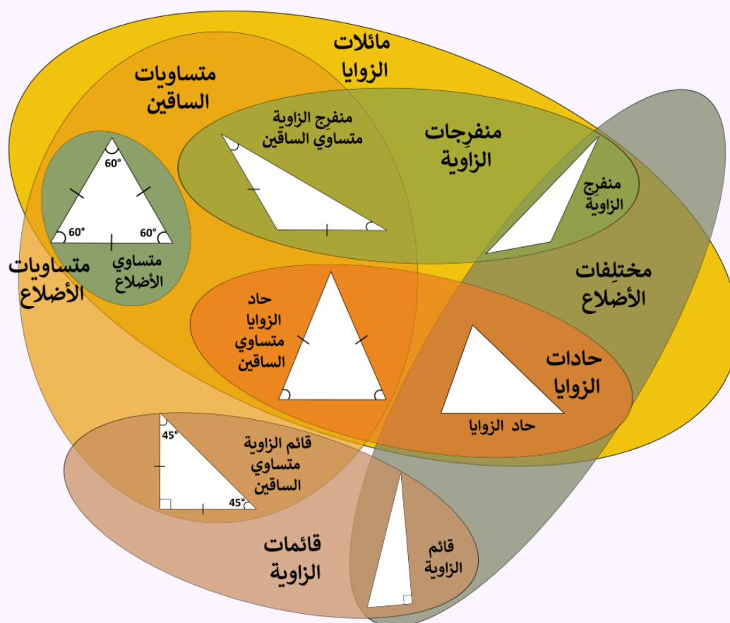
تصنيف المثلثات بمخطط قن
