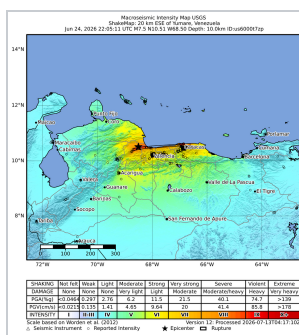
Karta makroseizmičkog intenziteta
