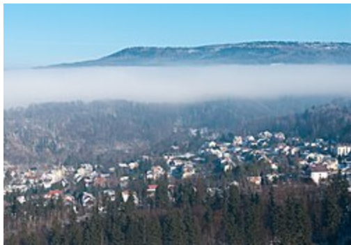
Warstwa mgły związana z inwersją , nad Kudową-Zdrojem
