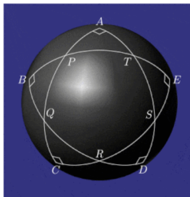
Przykładowe konfiguracje pentagrama mirificum
