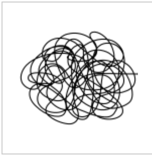
Chaos.svg 226 × 192; 11 KB
