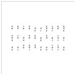
D2-Test.jpg 462 × 248; 18 KB
