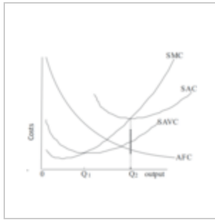
Avc atc mc.png 477 × 376; 24 KB
