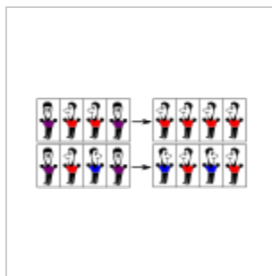
SznajdModelSketch.svg 740 × 317; 62 KB
